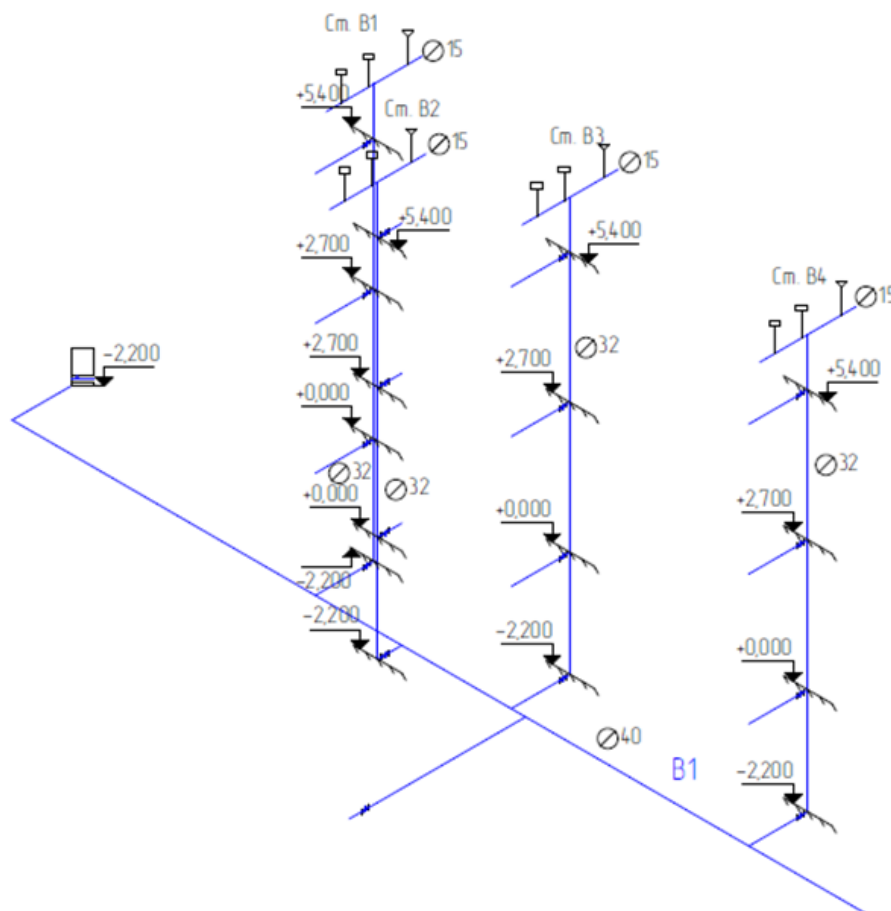
Аксонометрия системы внутреннего водопровода
